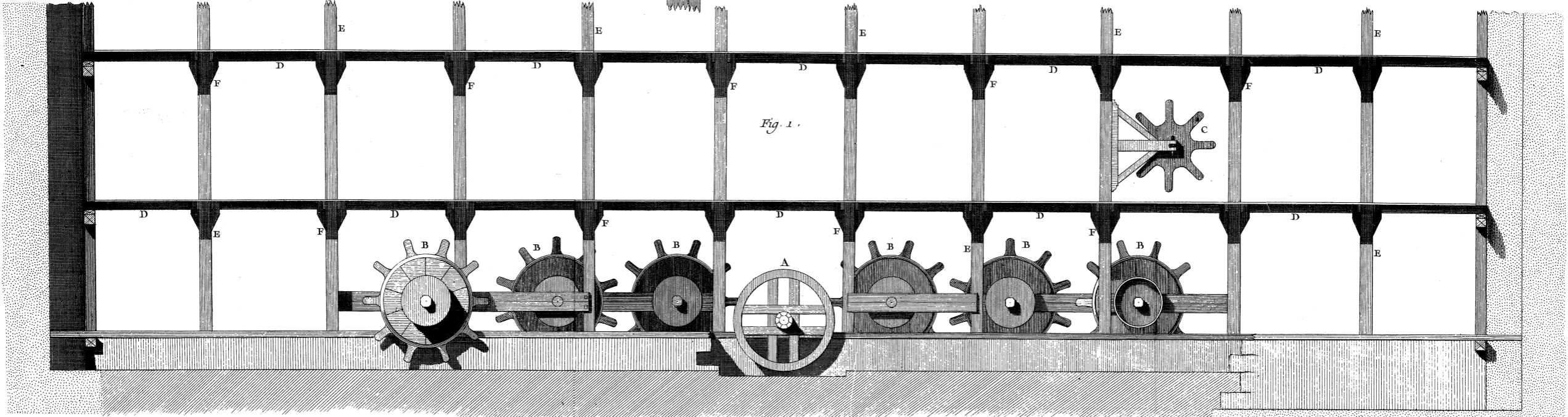
Machines de Théâtres, Coupe sur la largeur des deux premiers Planchers du dessous de la Salle de l'Opéra de Paris, avec différens Détails de Construction.
